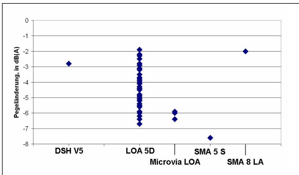
Abbildung 8: Erzielte Pegelminderung in Abhängigkeit von der neuen Fahrbahnoberfläche
