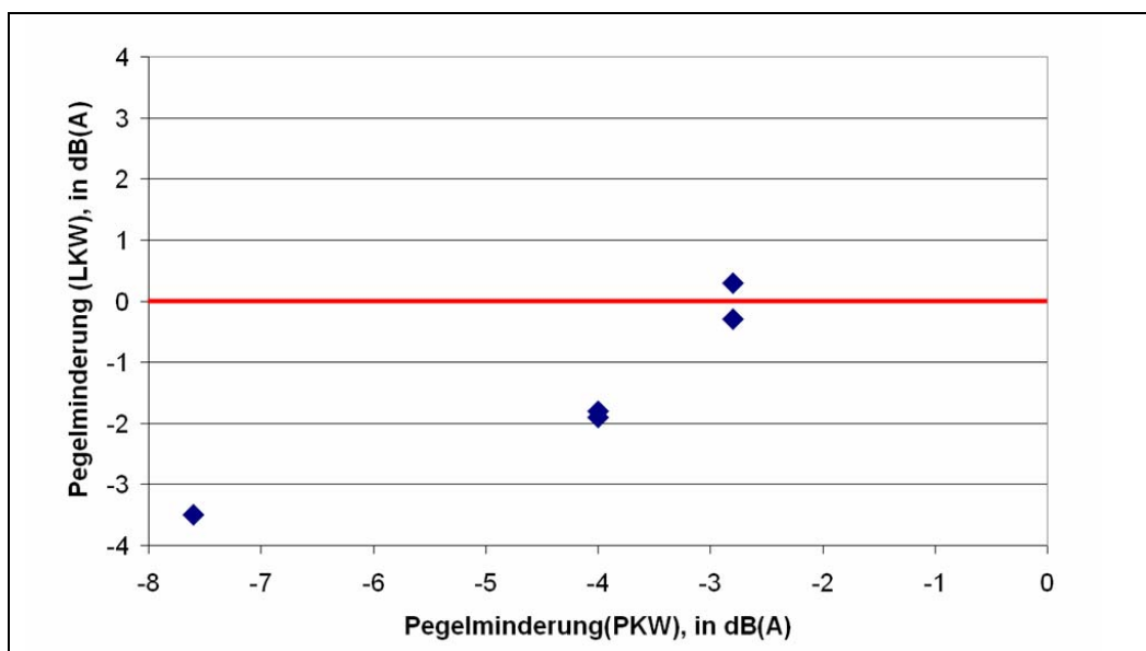
Abbildung 9: Durch den Einbau neuer Fahrbohnoberflächen erzielte Pegelminderung für PKW (x-Achse) und LKW (y-Achse). Die rote horizontale Linie markiert eine Minderung der LKW-Geräusche um 0 dB(A).
