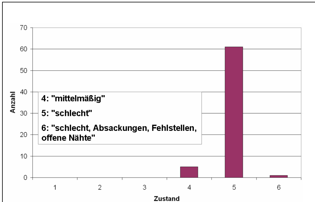
Abbildung 4: Zustand der ersetzten Fahrbahnoberflächen in einem Schulnotensystem (1-6) abgebildet.
