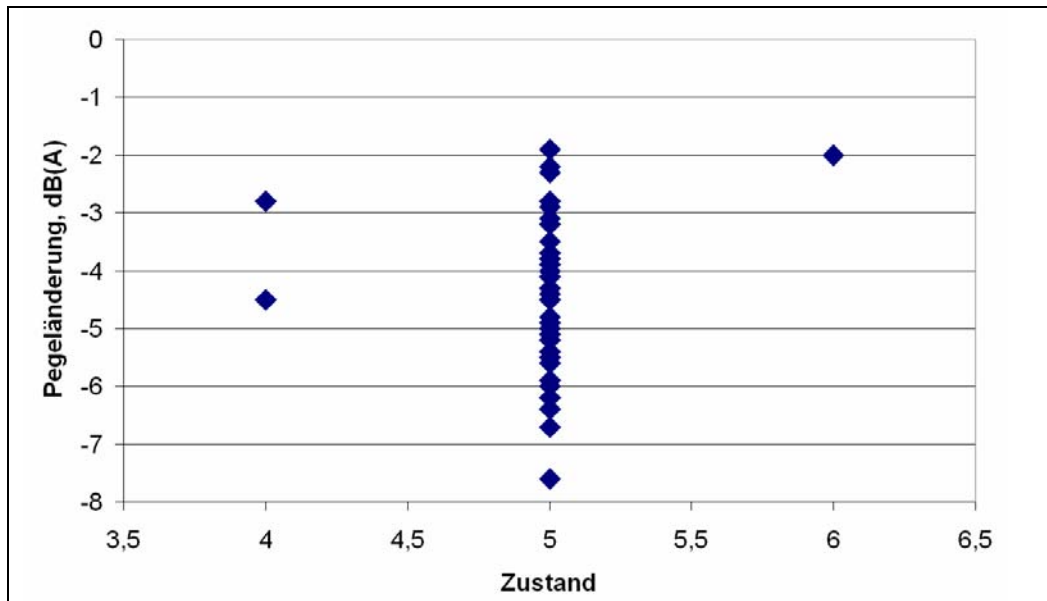
Abbildung 7: Erzielte Pegelminderung in Abhängigkeit vom Zustand der ursprünglichen Fahrbahnoberfläche.
